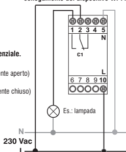
Schema elettrico di principio per il collegamento del dispositivo Wi-Fi
