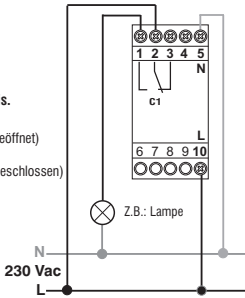
Hauptschaltplan für den Anschluss der WLAN-Vorrichtung
