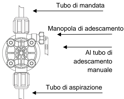
Modello di testata per pompa ad adescamento manuale, collegamenti alla testata della pompa in PVDF
